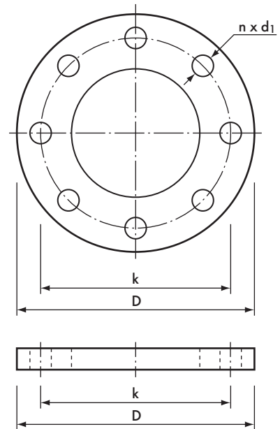
Рис. 2.1. Конструкция фланца
